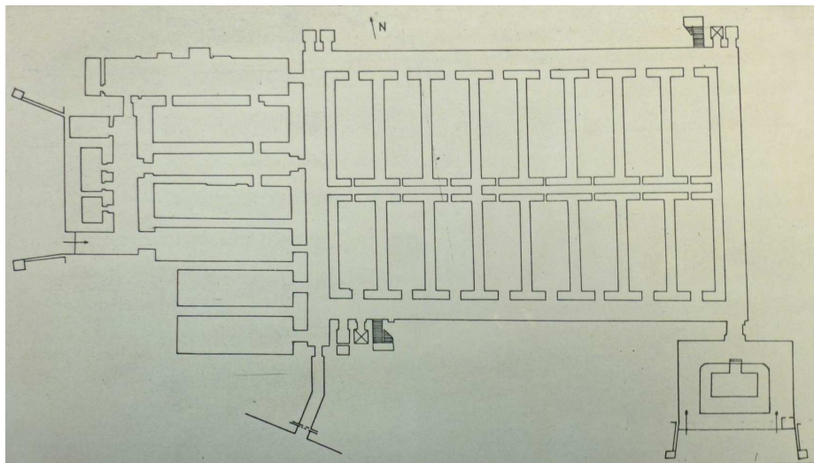
Rzut przyziemia wg karty ewidencyjnej obiektu (archiwum WUOZ Warszawa)
